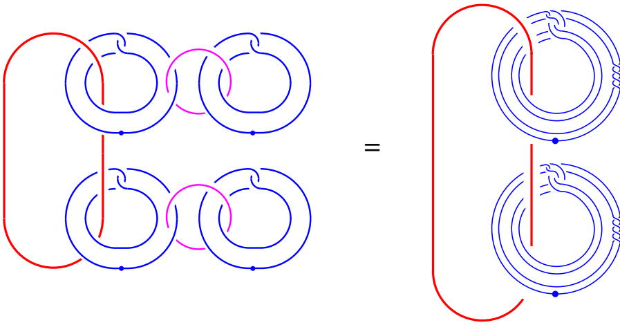
Figure 8: Another Type CH その1 (2階までの変形) p.396
